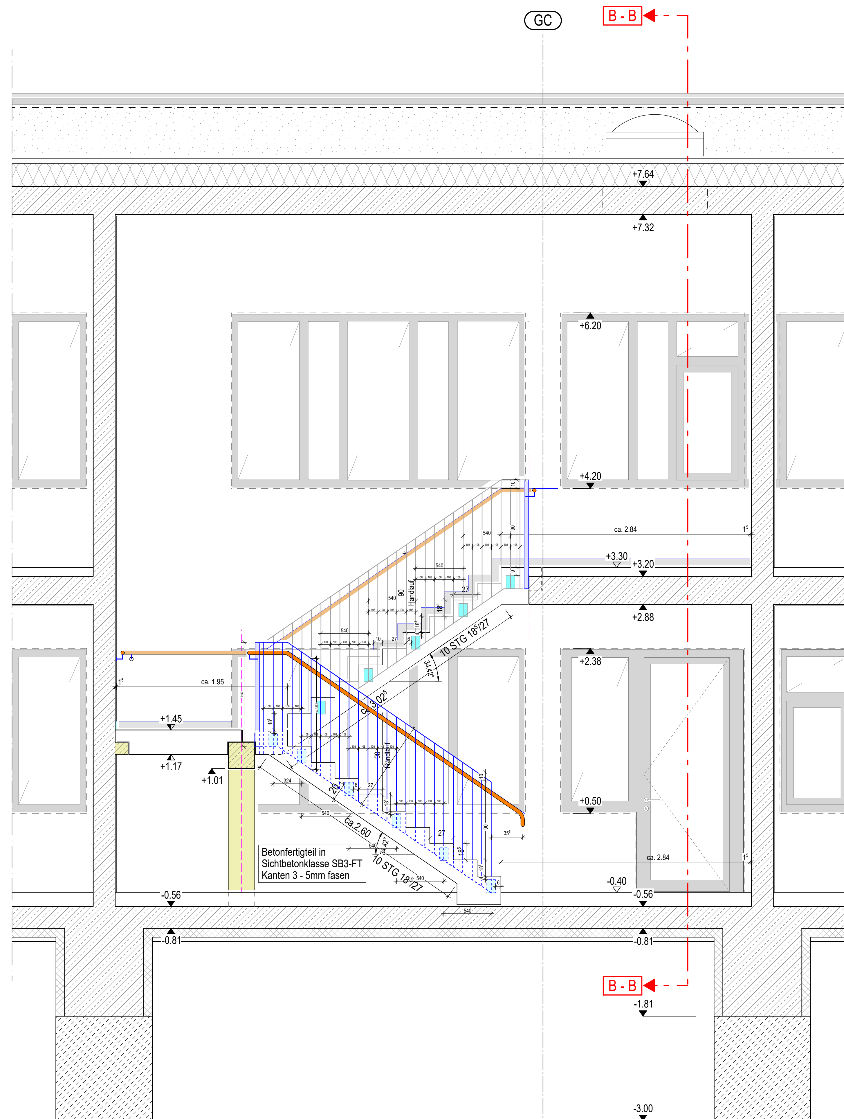
SCHNITT A - A
