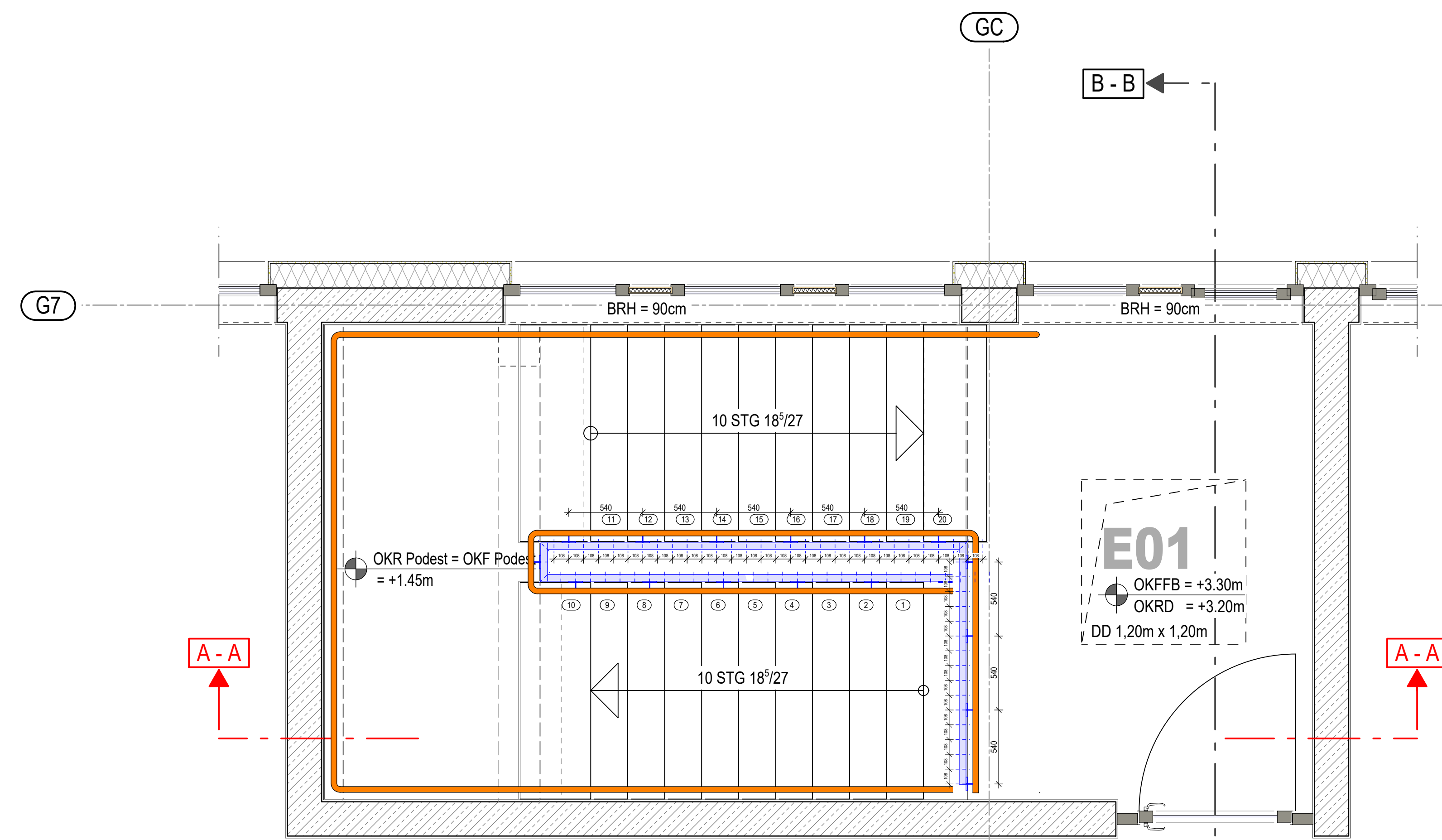
Grundrissausschnitt 1. OBERGESCHOSS
