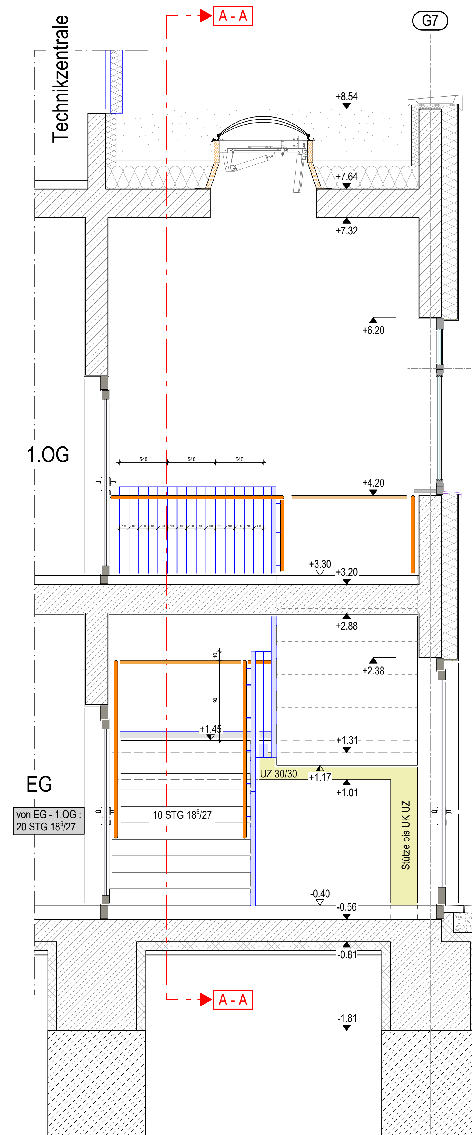
SCHNITT B - B
